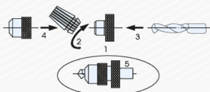
1 ปรับตำแหน่งของดอกสว่าน Set the position of the drill bit
