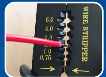
การปอกสาย STRIPPING
